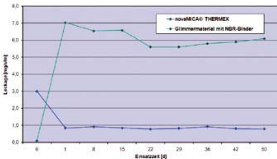
» 3 Warmleckage – Leckage unter Temperatur nach Langzeitlagerung bei 500 °C, Leckagebestimmung bei 5 bar in Anlehnung an DIN 28090-2
