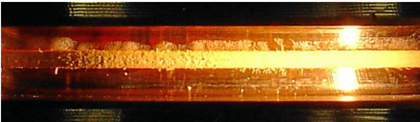
Bild 5 Spalt mit Spray nach 30 Sekunden 6 bar
