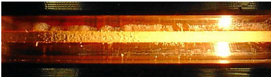
Bild 5 Spalt mit Spray nach 30 Sekunden 6 bar
