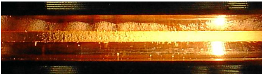
Bild 6 Spalt mit Spray nach 180 Sekunden 6 bar
